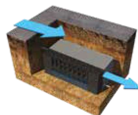
Regulacja przepływu (opóźnienie odprowadzenia wody burzowej)
